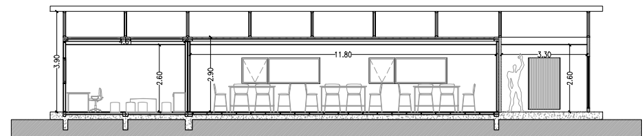
Corte Transversal
