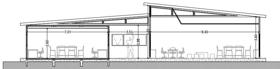
Corte Transversal
