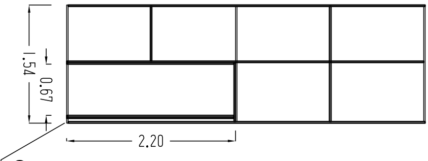
ELEVACION FRONTAL Estructura Interna
