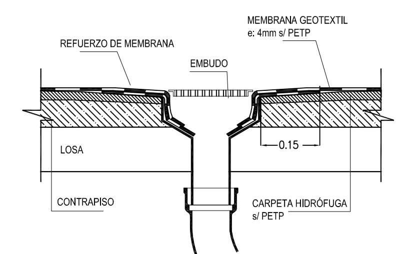
DETALLE ENCUENTRO EMBUDO
