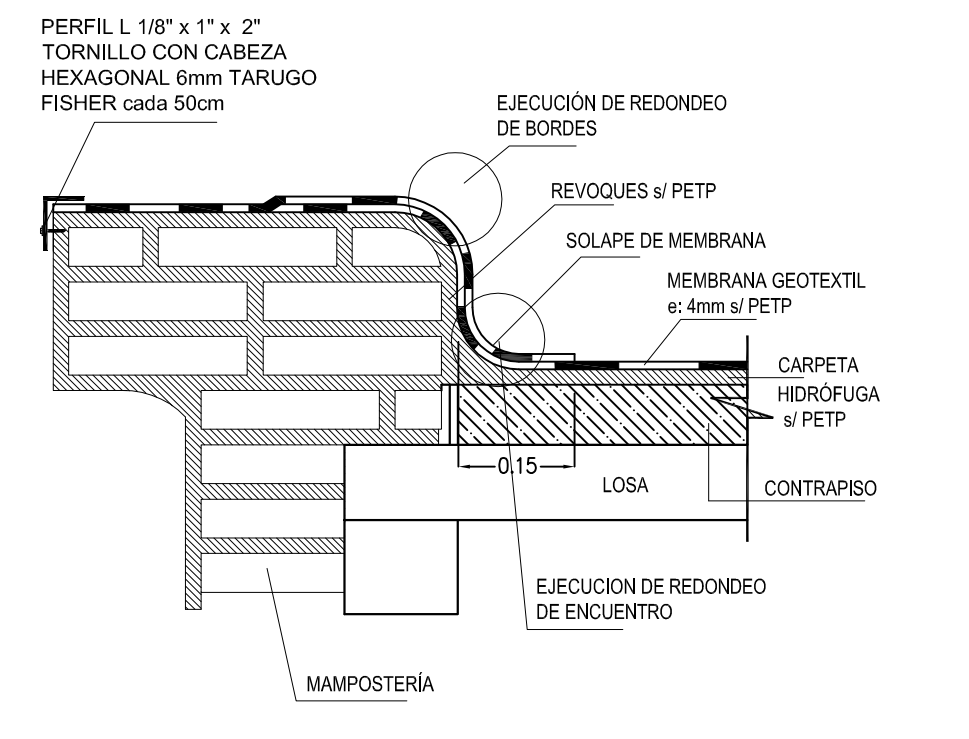
DETALLE TERMINACION EN BORDES
