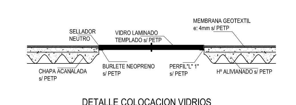
DETALLE COLOCACION VIDRIOS
