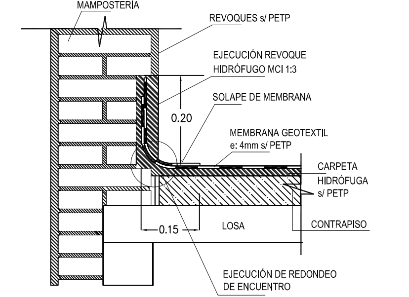
DETALLE ENCUENTRO MAMPOSTERIA
