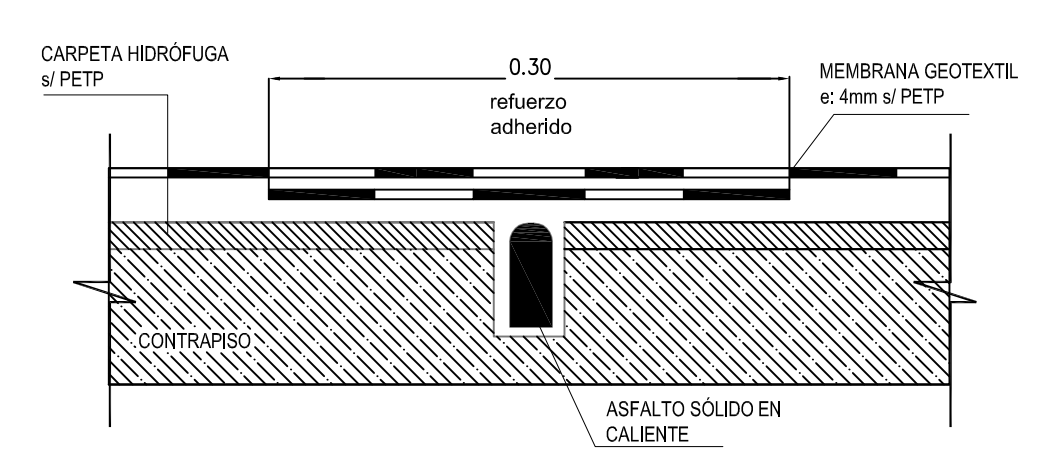
DETALLE DE JUNTA DE DILATACION
